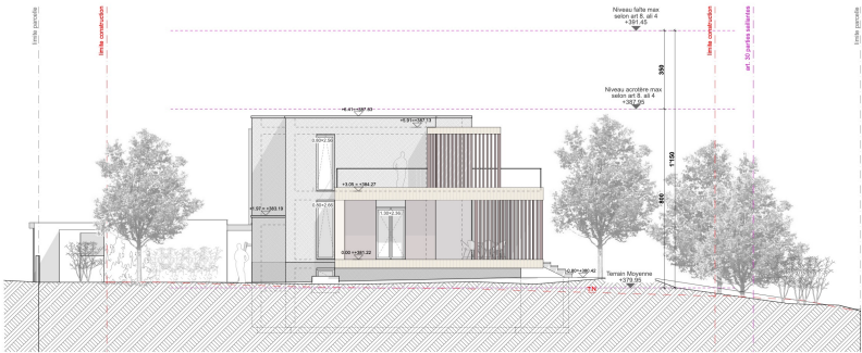
FACADE OUEST
