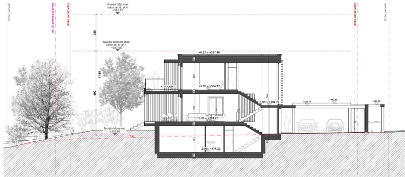
COUPE A
