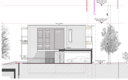
FACADE NORD
