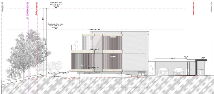
FACADE EST
