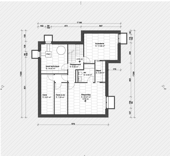
SOUS-SOL
