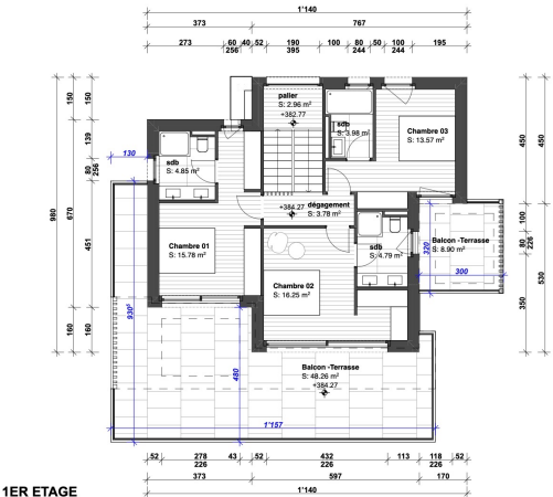
1ER ETAGE
