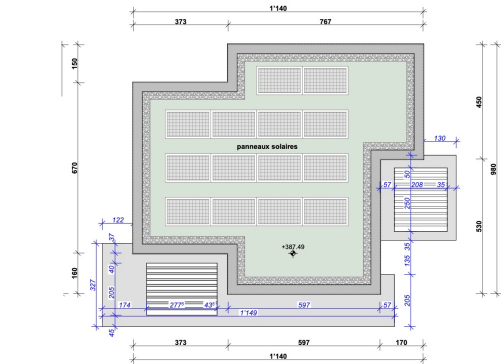
TOITURE
