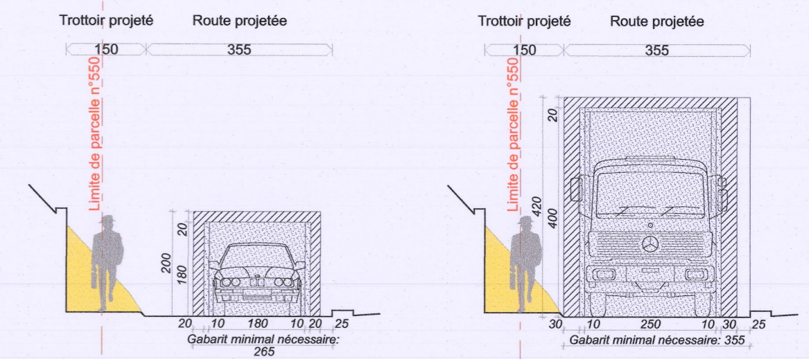
Coupe 1
