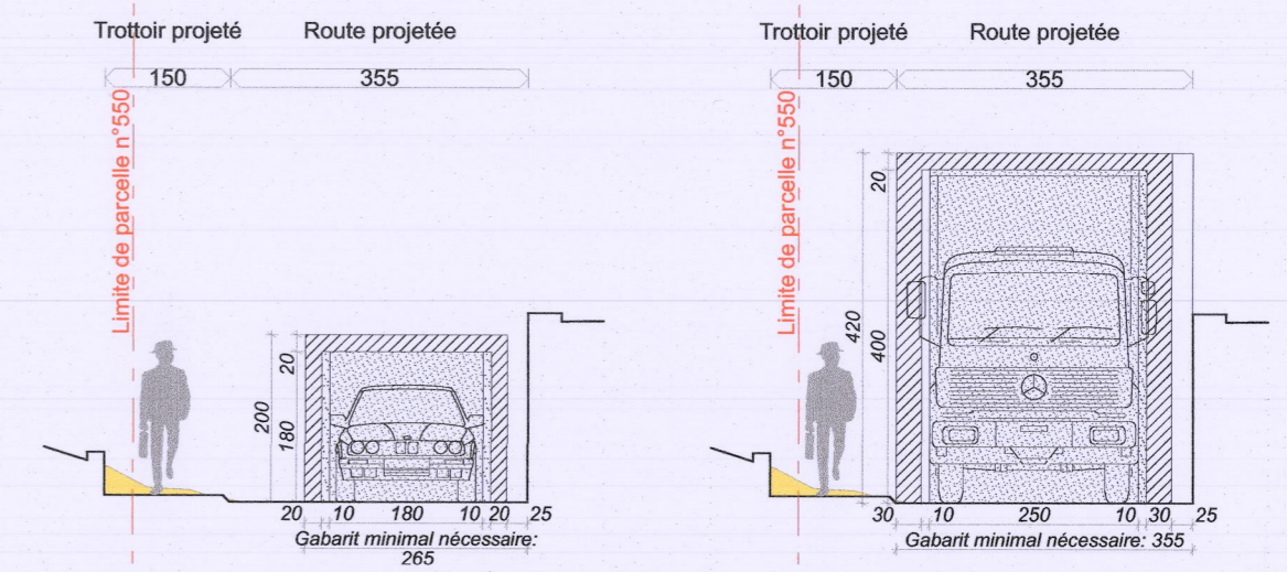
Coupe 2
