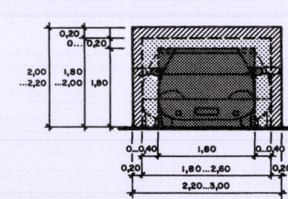
Fig. 3: Gabarit des voitures de tourisme
