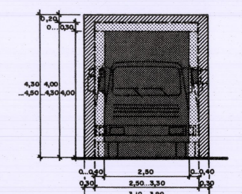
Fig. 4: Gabarit des poids lourds, bus et autocars
