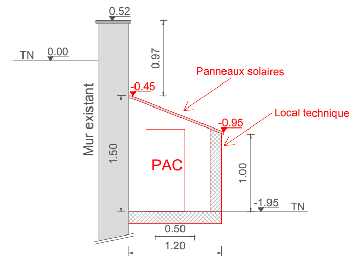
Coupe CC'
